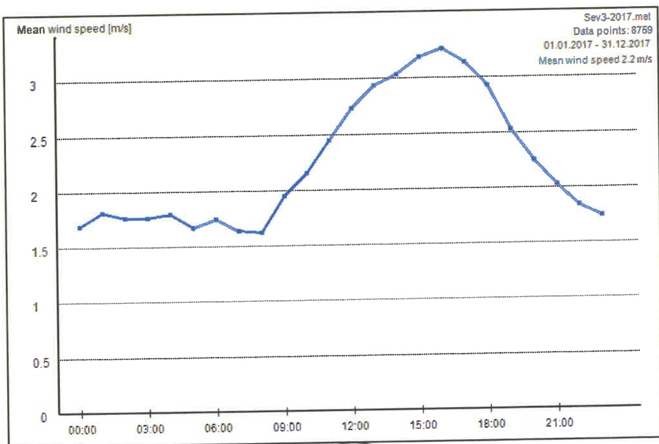
Figura C.10.4.1. – Variația zilnică a vitezei vântului predominant în anul 2017 la stația meteorologică Drobeta – Turnu Severin
