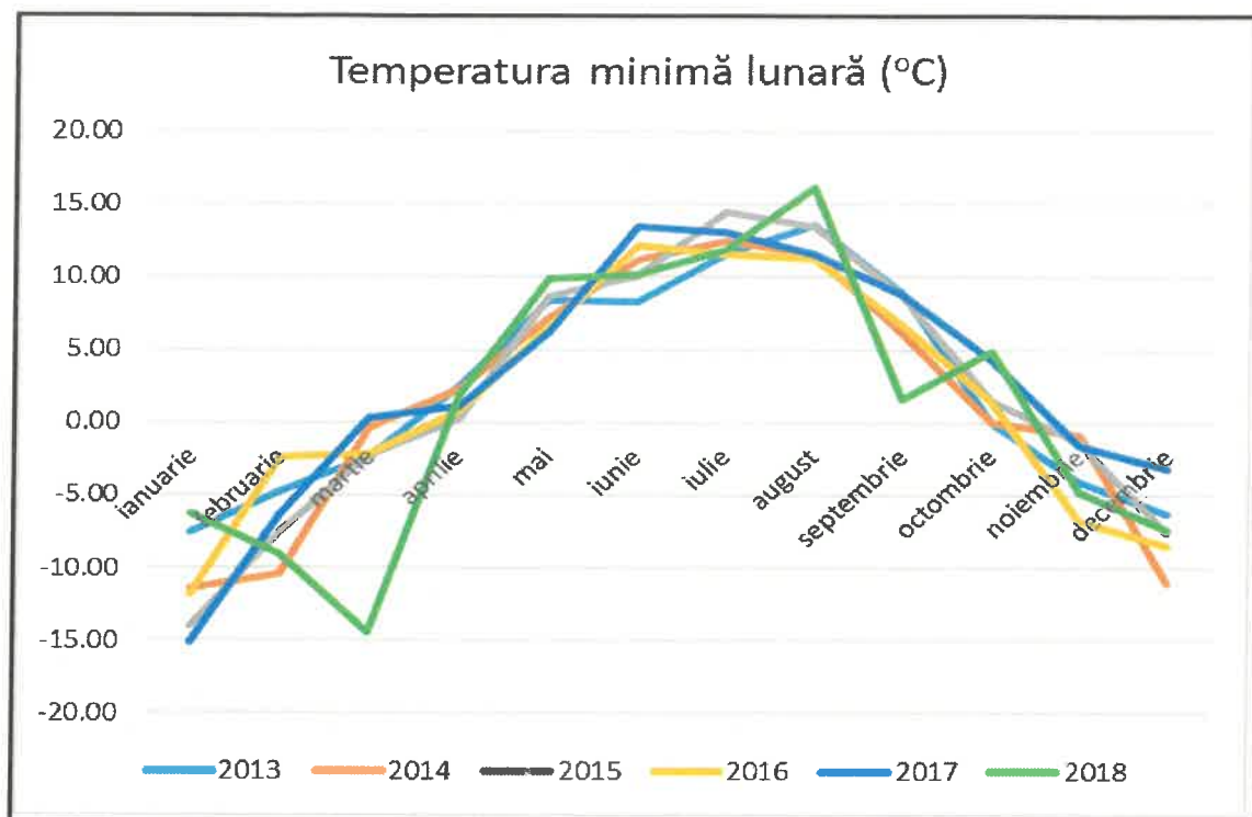
Figura B.4.5. – Evoluția temperaturilor minime lunare la stația Drobeta-Turnu-Severin în perioada 2013-2018
