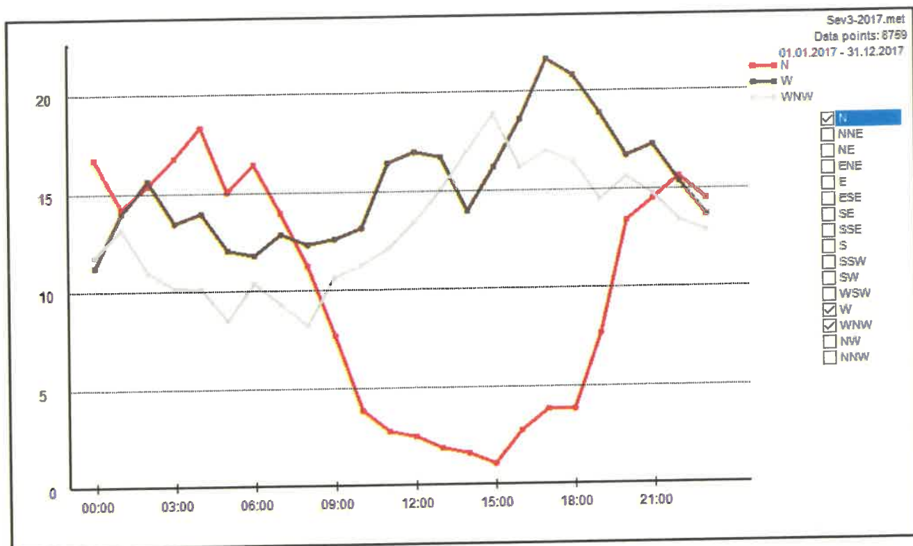
Figura C.10.3.1. – Variația zilnică a direcției vântului în anul 2017 la stația meteorologică Drobeta – Turnu Severin
