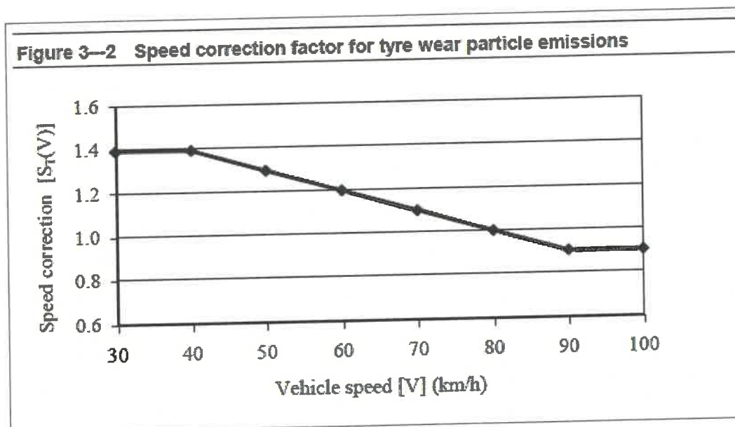
Figura D.6.1.3.1. – Variația cu viteza emisiilor rezultate din uzura pneurilor (după Ghidul EMEP v. 2016)
