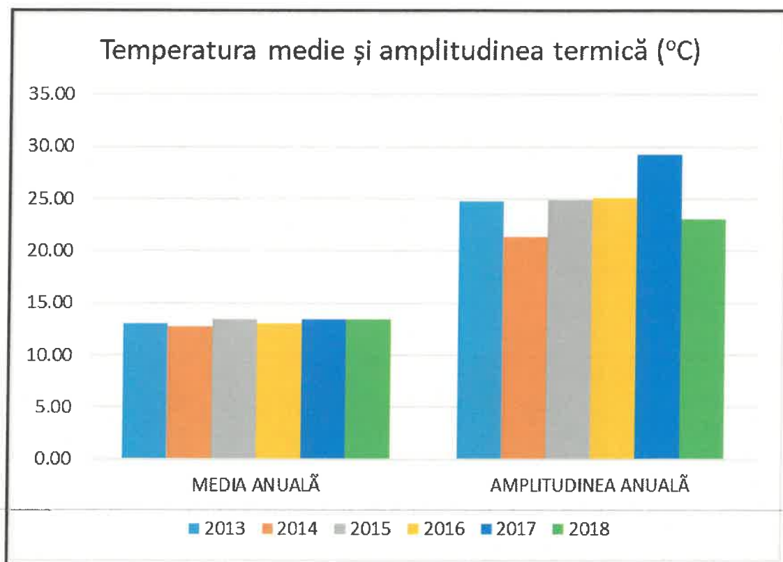
Figura B.4.2. – Evoluția temperaturilor medii anuale și amplitudinii termice la stația Drobeta - Turnu-Severin în perioada 2013-2018
