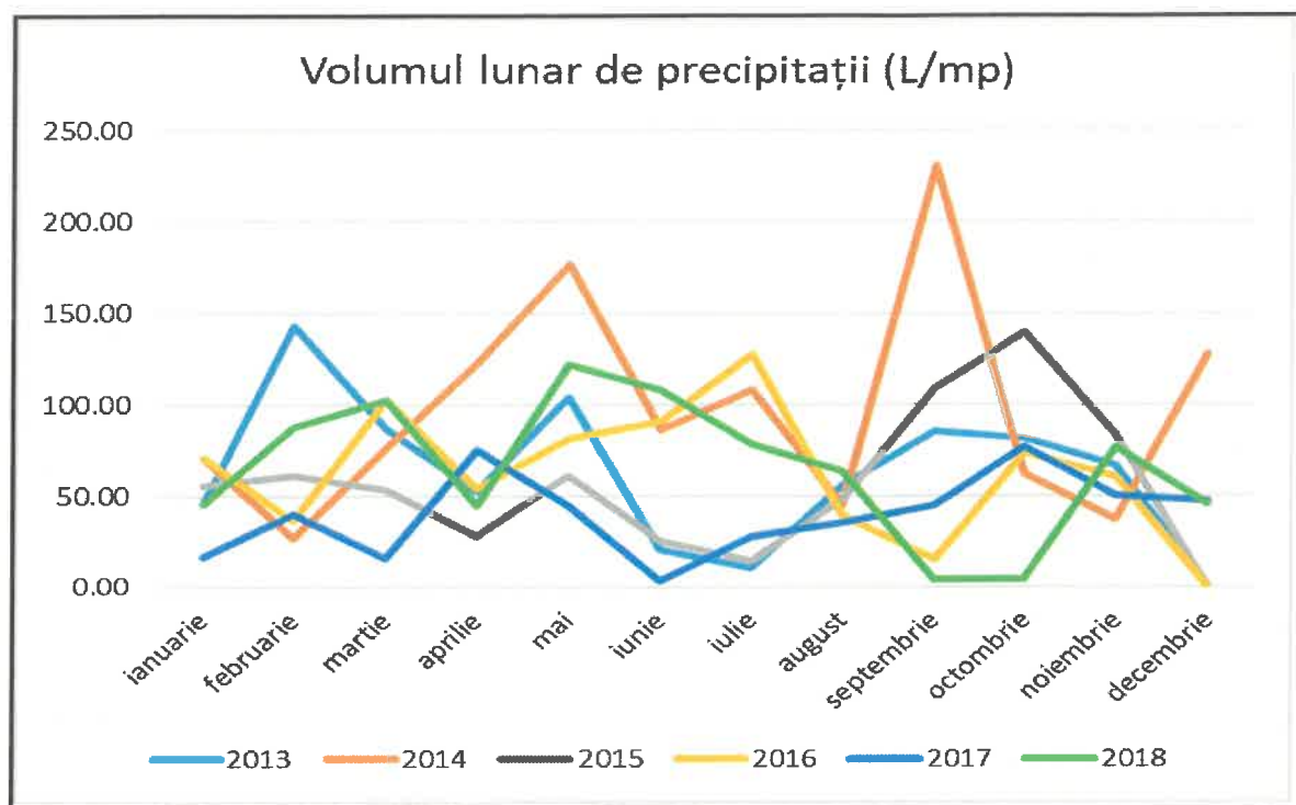
Figura B.4.7. – Evoluția precipitațiilor lunare la stația Drobeta-Turnu-Severin în perioada 2013-2018
