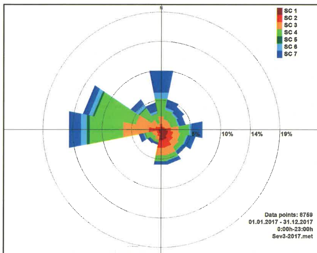
Figura C.10.2.1. Stabilitatea vântului în anul 2017 la stația meteorologică Drobeta – Turnu Severin
