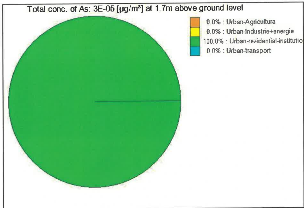
Anexa D.9.3.1.0 – Repartiția surselor de As în mediul urban din zona Mehedinți în anul de proiecție
