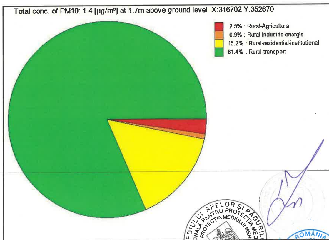
Anexa C.6.3.2.0 – Repartiția surselor de PM10 în mediul rural din zona Mehedinți în anul de proiecție
