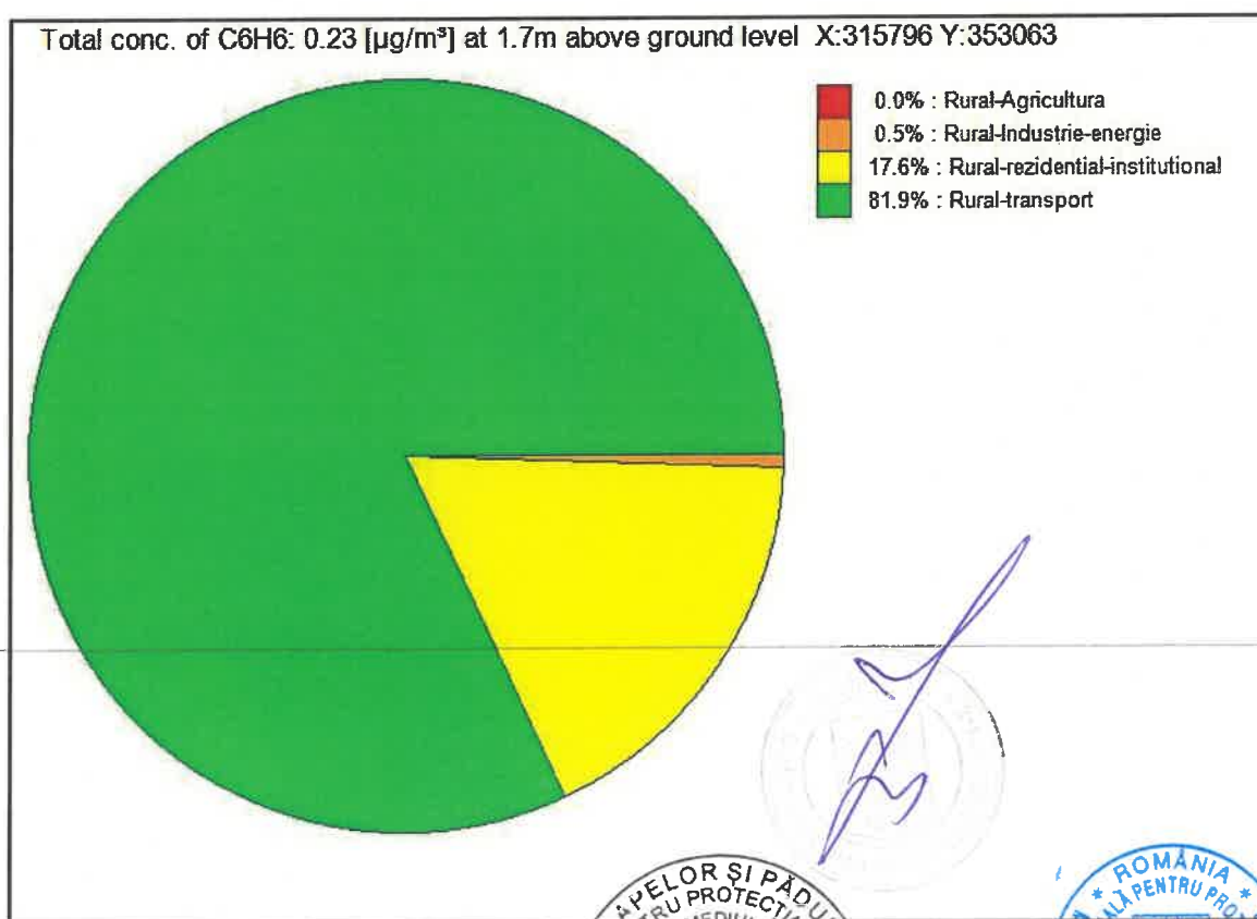
Anexa D.5.3.2.0 – Repartiția surselor de benzen în mediul rural din zona Mehedinți în anul de proiecție
