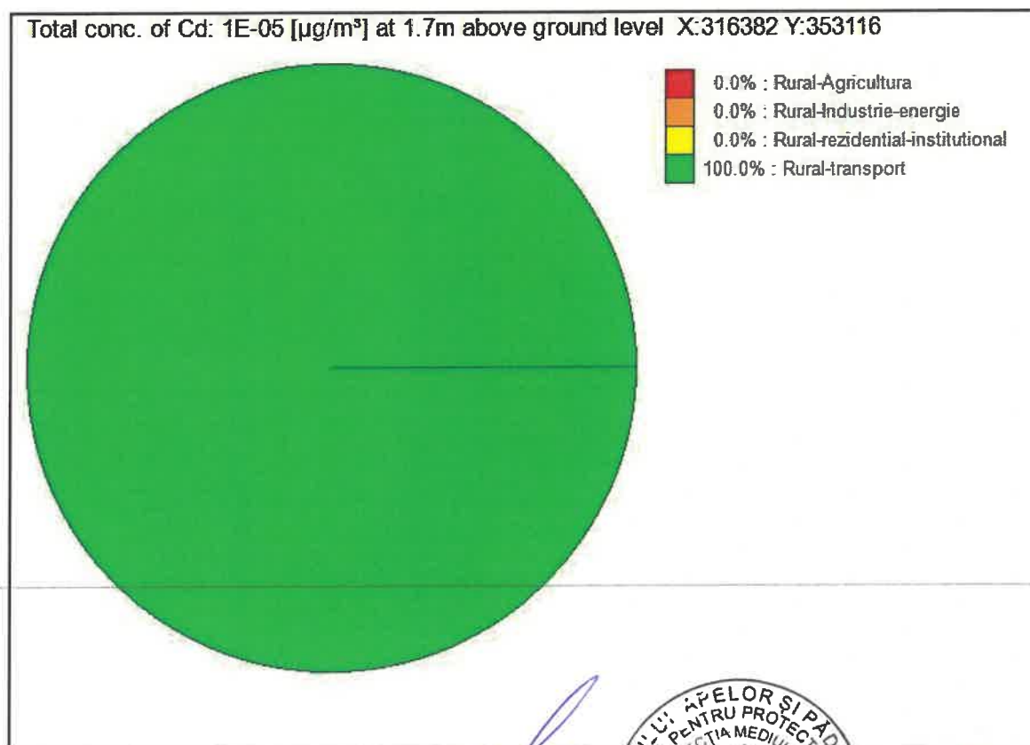
Anexa D.10.3.2.0 – Repartiția surselor de Cd în mediul rural în zona Mehedinți în anul de proiecție
