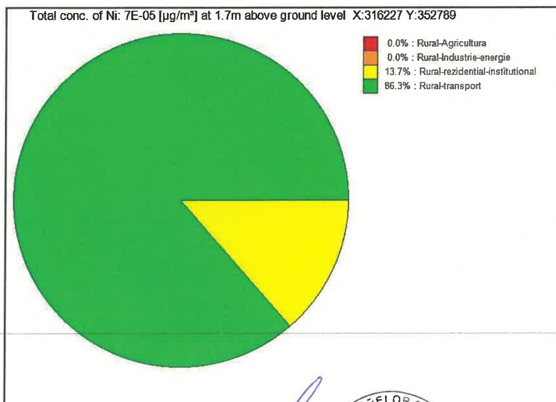
Anexa D.11.3.2.0 – Repartiția surselor de Ni în mediul rural din zona Mehedinți în anul de proiecție
