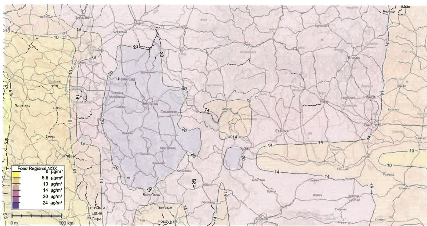
Anexa R.3.1.1.0 – Fond regional NOx pentru județul Mehedinți în anul de referință
