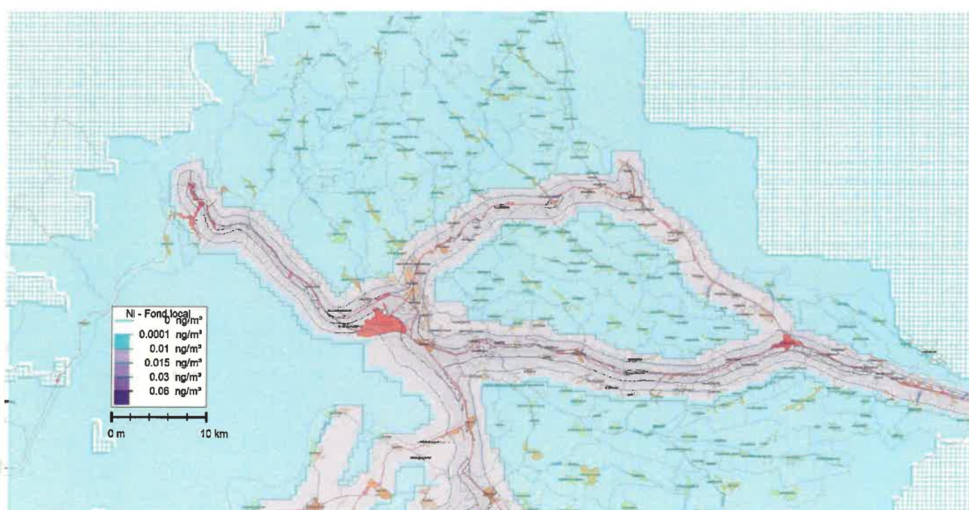
Anexa D.11.2.1.0 – Dispersia Ni în mediul rural din zona Mehedinți în anul de proiecție
