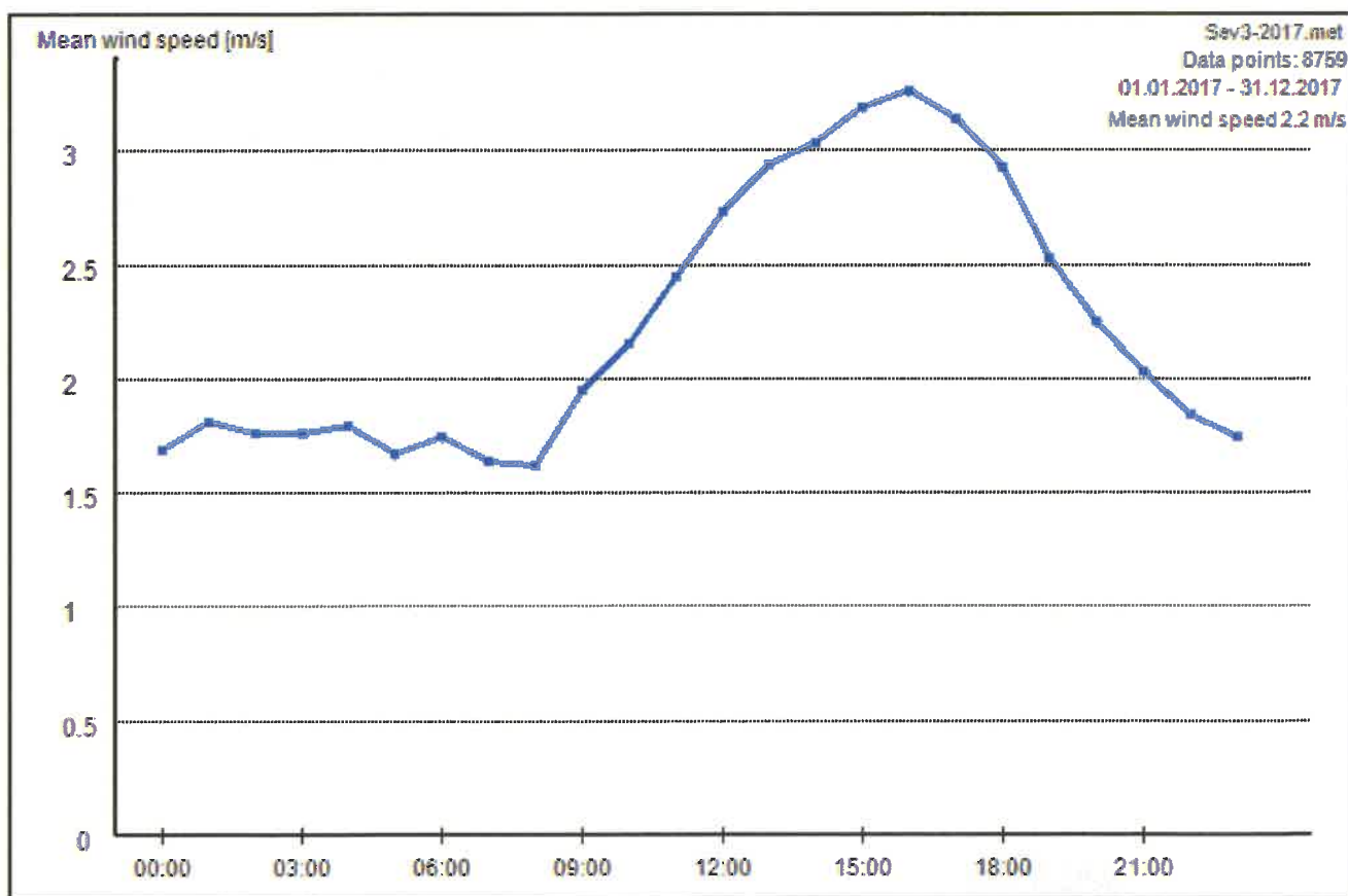
Figura C.10.4.1 – Variația zilnică a vitezei vântului medii în anul 2017 la stația meteorologică Drobeta – Turnu Severin
