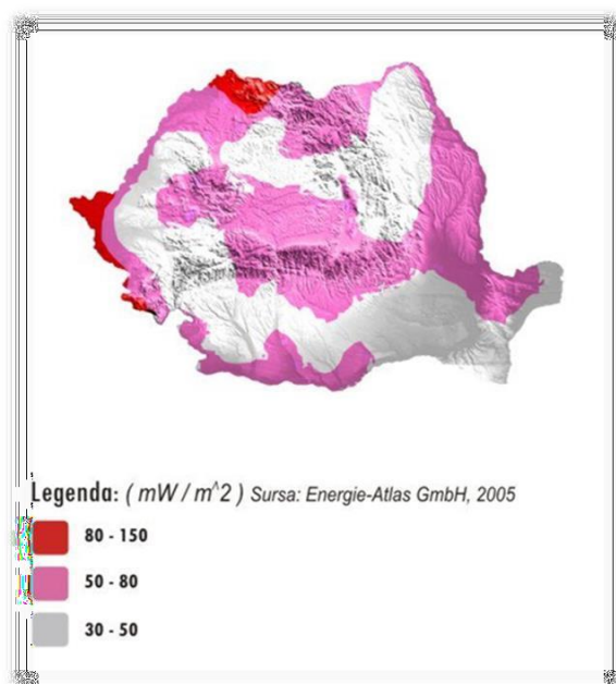
Fig. nr. 33 — Zone cu potențial geotermal
