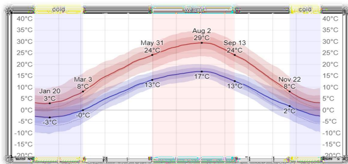
Fig.nr. 2 — Temperaturi medii lunare
